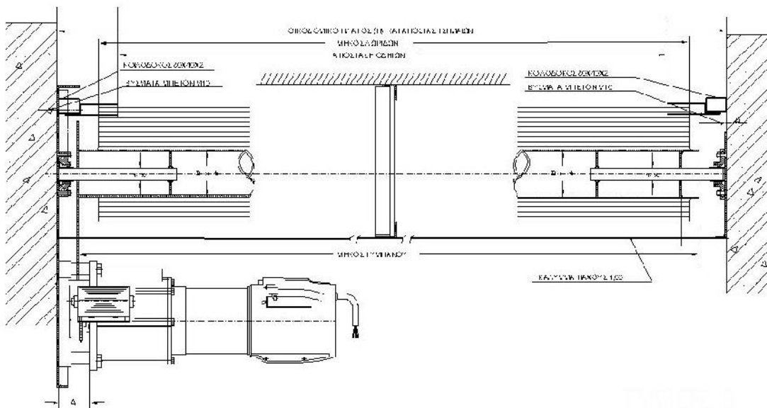
ΠΥΡΑΝΤΟΧΟ ΡΟΛΟ - ΕΣΩΤΕΡΙΚΗΣ ΤΟΠΟΘΕΤΗΣΗΣ (ΟΡΙΖΟΝΤΙΑ ΤΟΜΗ)
