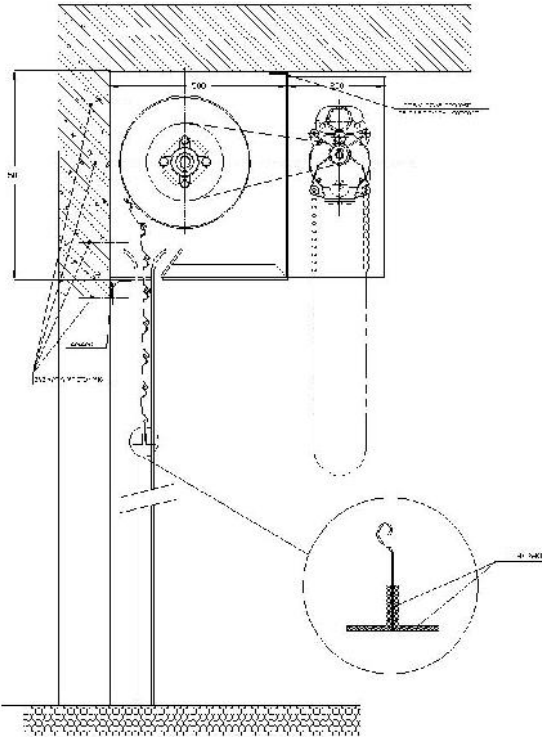
ΠΥΡΑΝΤΟΧΟ ΡΟΛΟ - ΕΞΩΤΕΡΙΚΗΣ ΤΟΠΟΘΕΤΗΣΗΣ (ΚΑΘΕΤΗ ΤΟΜΗ)
