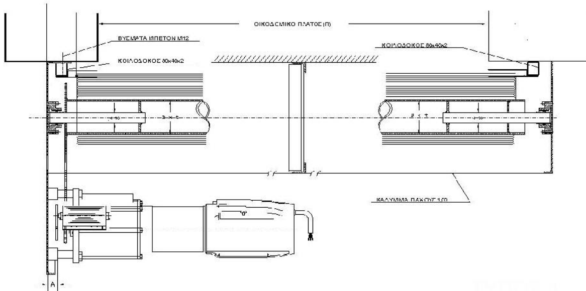
ΠΥΡΑΝΤΟΧΟ ΡΟΛΟ - ΕΞΩΤΕΡΙΚΗΣ ΤΟΠΟΘΕΤΗΣΗΣ (ΟΡΙΖΟΝΤΙΑ ΤΟΜΗ)
